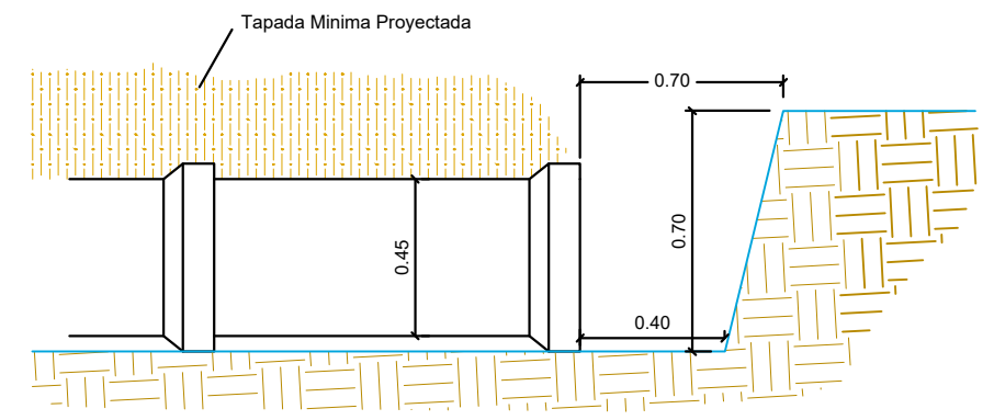
DETALLES ZANJEO PROYECTADO
