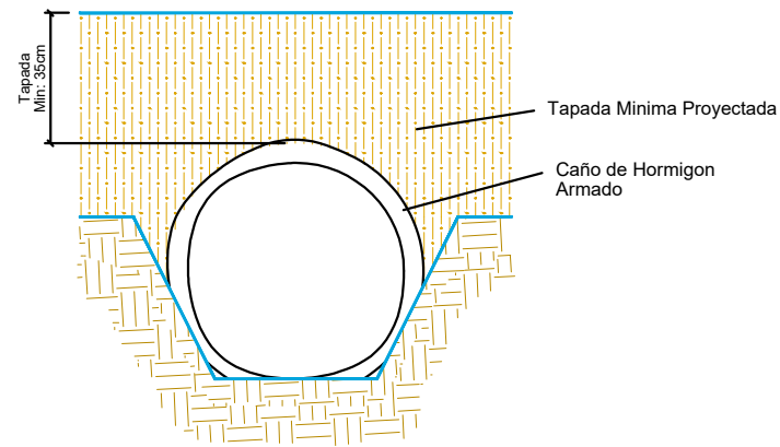
TAPADA DE CAÑO DE HORMIGON ARMADO EN CALLE DE TIERRA
