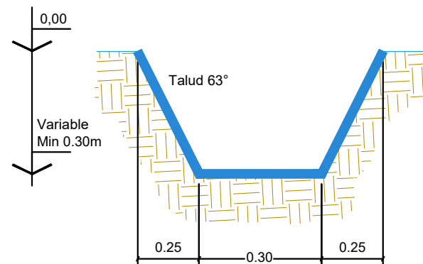
Tirante de Canal
