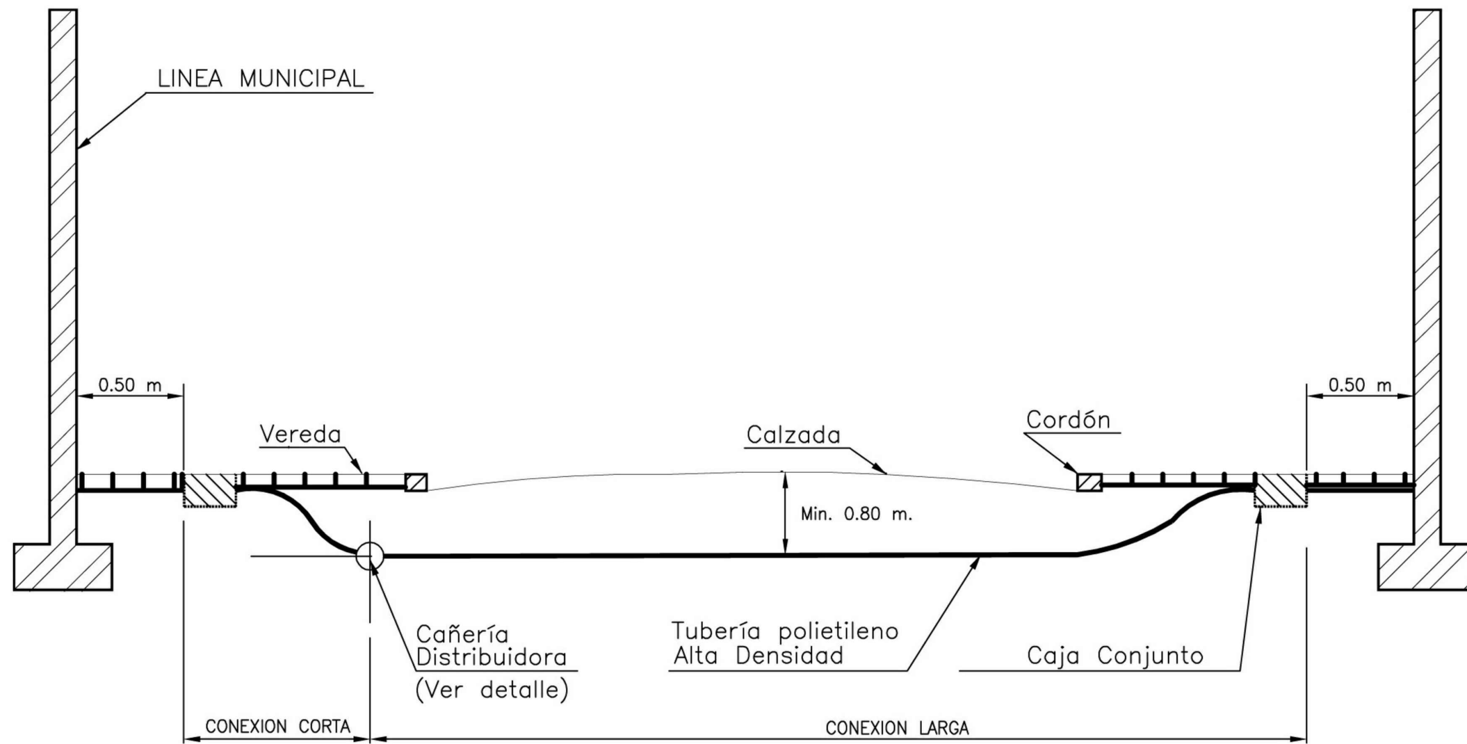
DETALLE CONEXION CAÑERIA DISTRIBUIDORA
