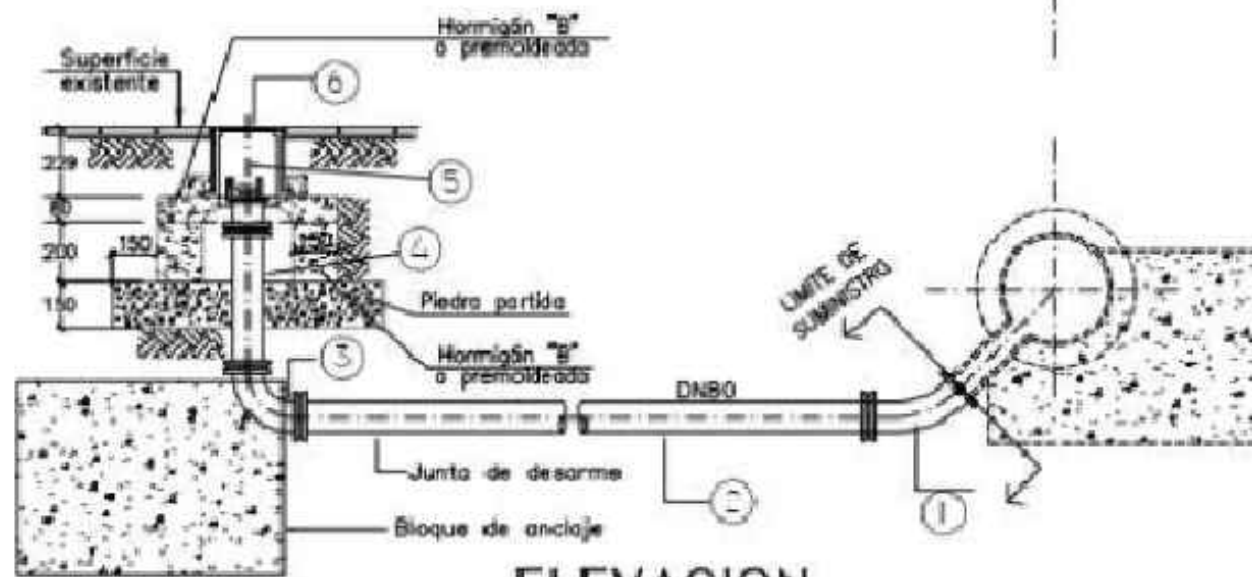
ELEVACION
