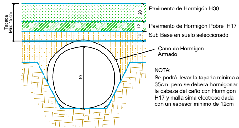
TAPADA DE CAÑO DE HORMIGON ARMADO EN PAVIMENTO DE HORMIGON RIGIDO - EN EJE DE CALLE
