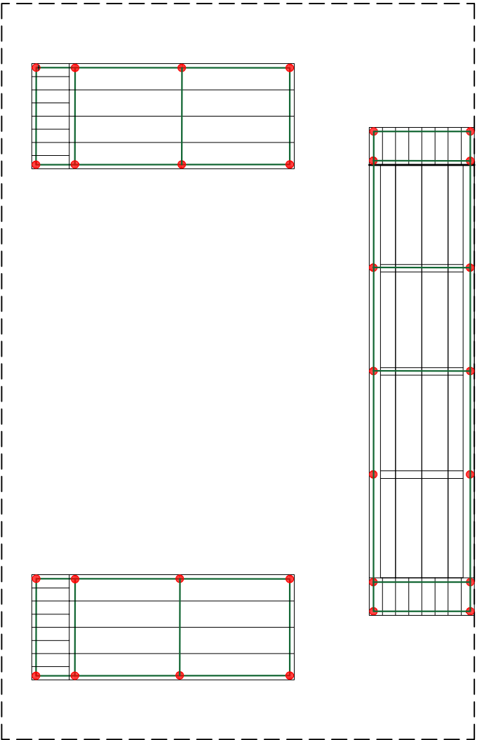
PILOTINES Y VIGA DE ENCADENADO GRADAS
