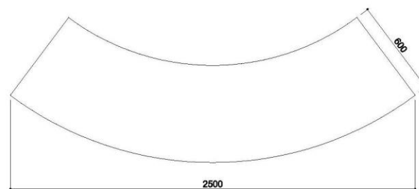
VISTA SUPERIOR - Curvo sin respaldo. 250 x 60 x 43h
