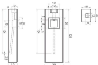
BEBEDERO RECTANGULAR
