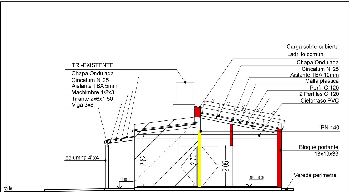
CORTE A-A
