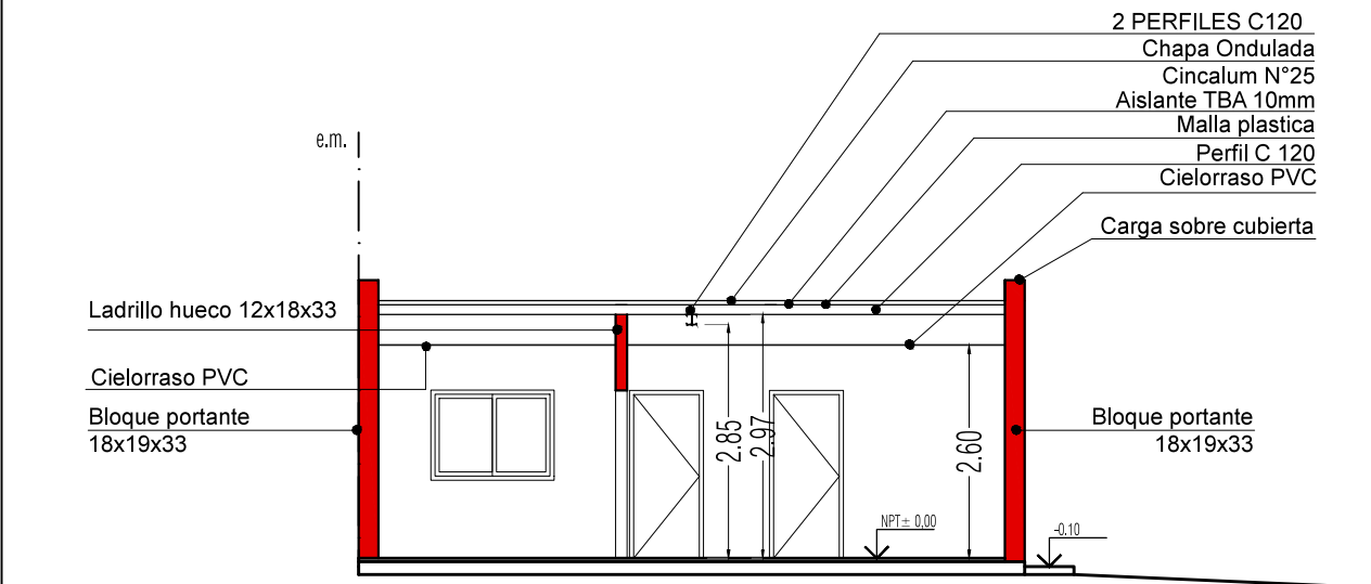
CORTE B-B
