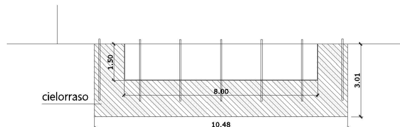
PLANTA MARQUESINA DEFINITIVA
