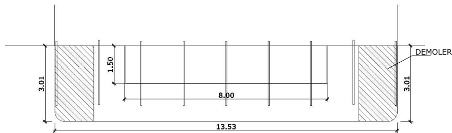
PLANTA ACTUAL MARQUESINA
