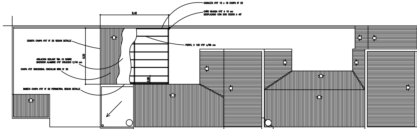
PLANTA DE TECHOS
