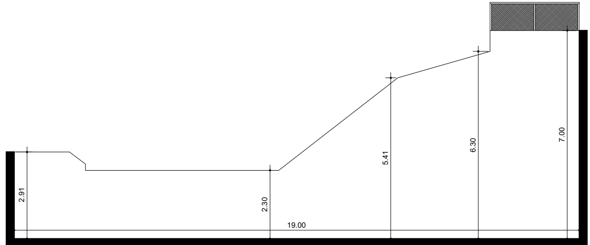
CORTE A-A ESTADO ACTUAL
