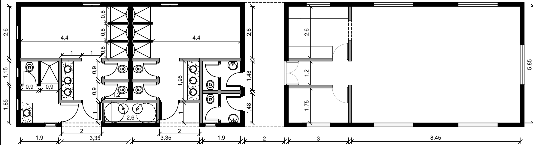
PLANTA ARQUITECTURA 1:100
