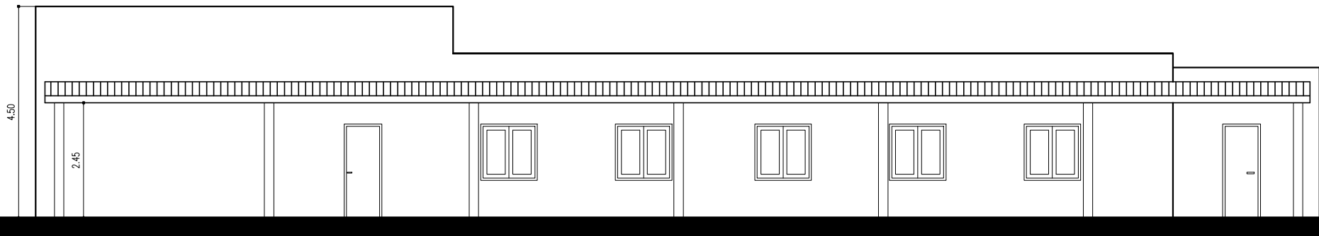
VISTA LONGITUDINAL
