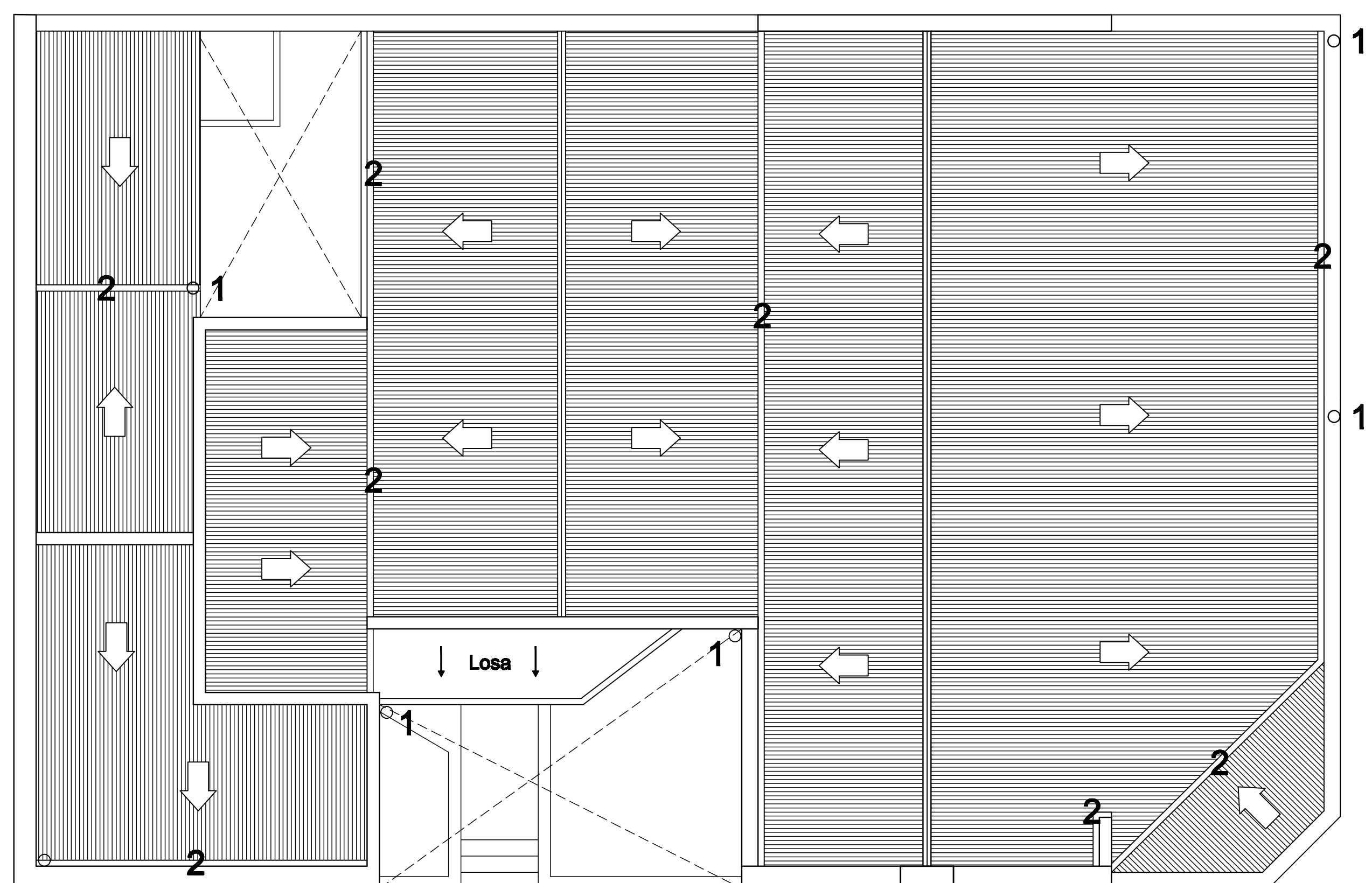
PLANTA DE TECHOS (a construir) Esc. 1:100
