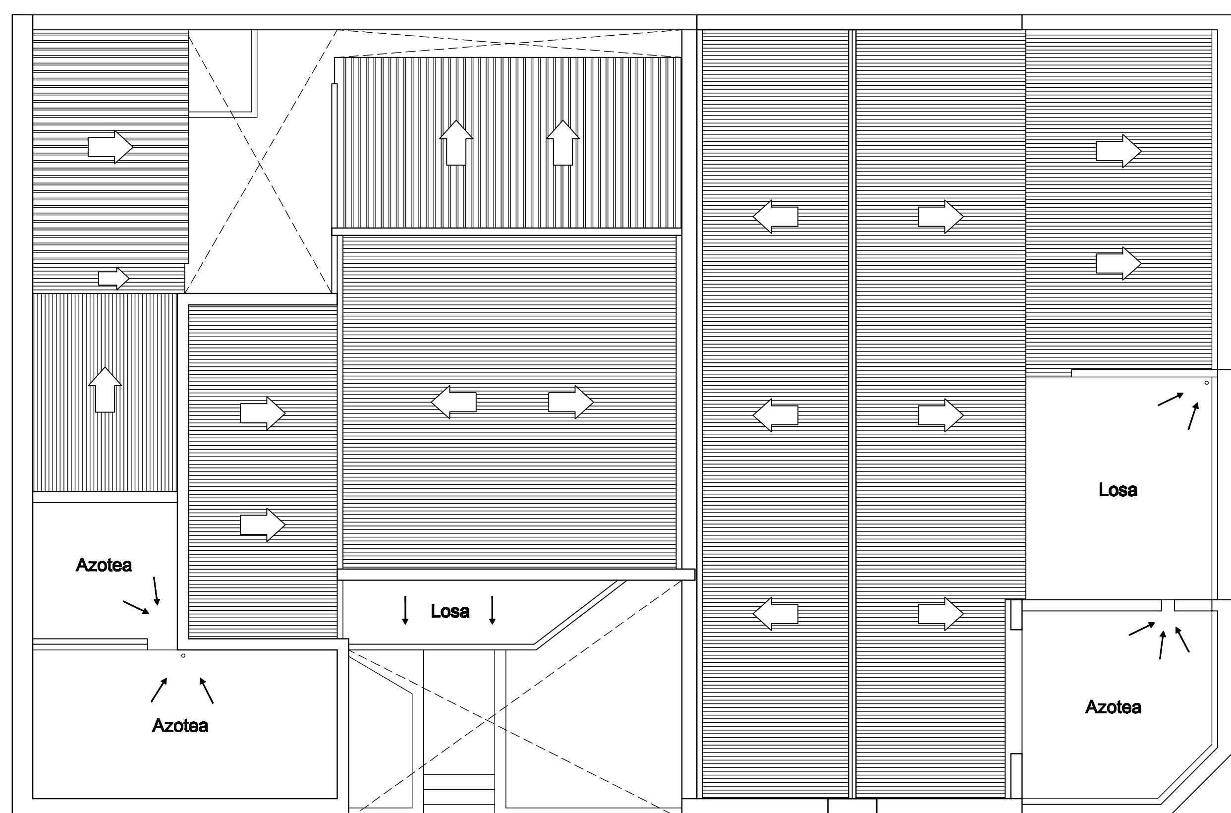
PLANTA DE TECHOS (existente) Esc. 1:100
