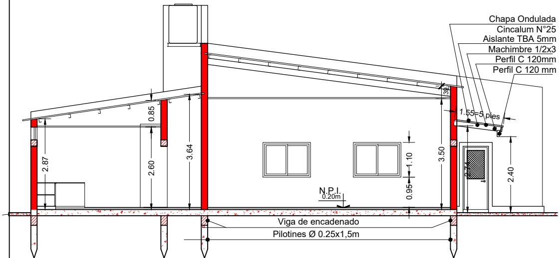
CORTE B-B
