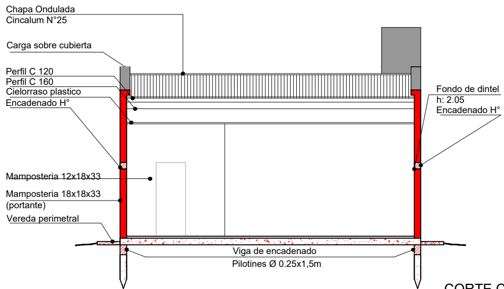
CORTE C-C
