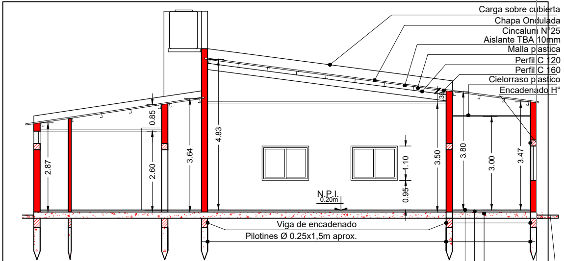
CORTE B-B
