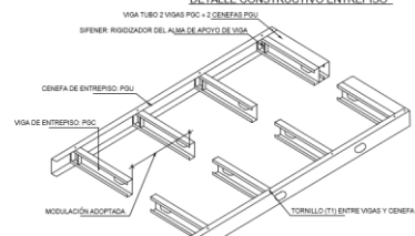
DETALLE CONSTRUCTIVO ENTREPISO.
