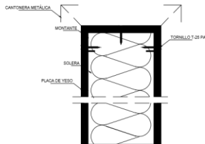
DETALLE CONSTRUCTIVO PARED DE DURLOCK.
