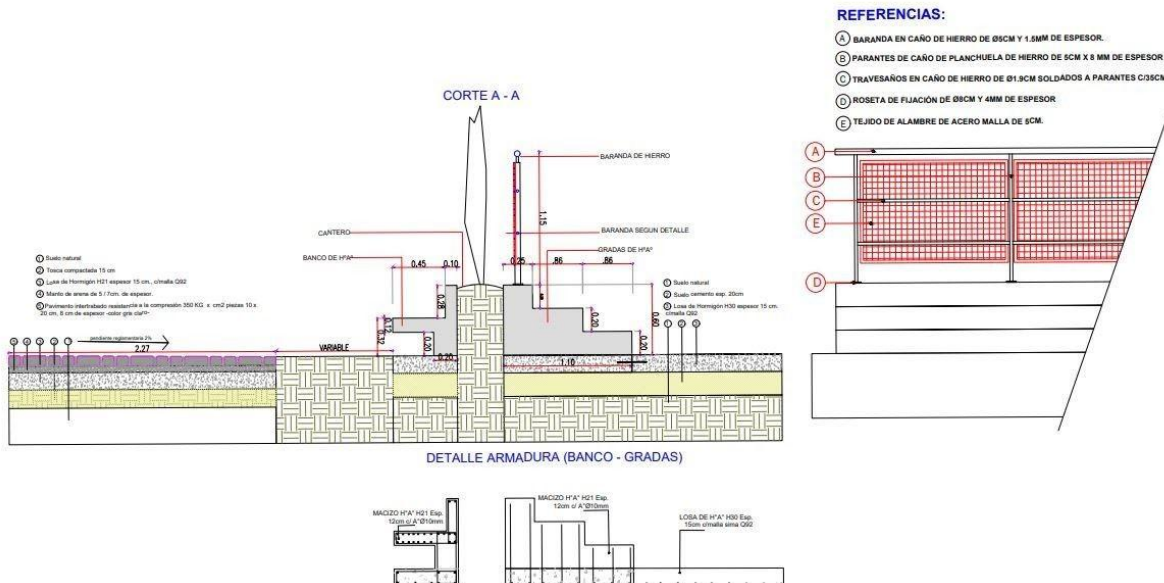
Plano de detalles constructivos de obra.
