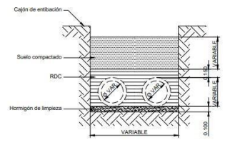
DETALLE DE EXCAVACIÓN CONDUCTO CIRCULAR DOBLE ESCALA 1:25
