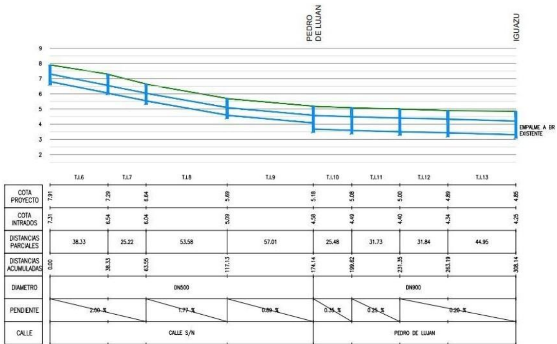
PERFIL 1 Escala Horizontal 1:1000 Escala Vertical 1:100
