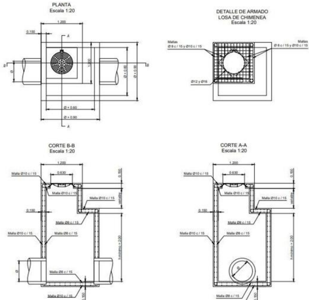
Arriba: Detalle cámara de inspección cloacal Abajo: | Boca de registro cloacal.
