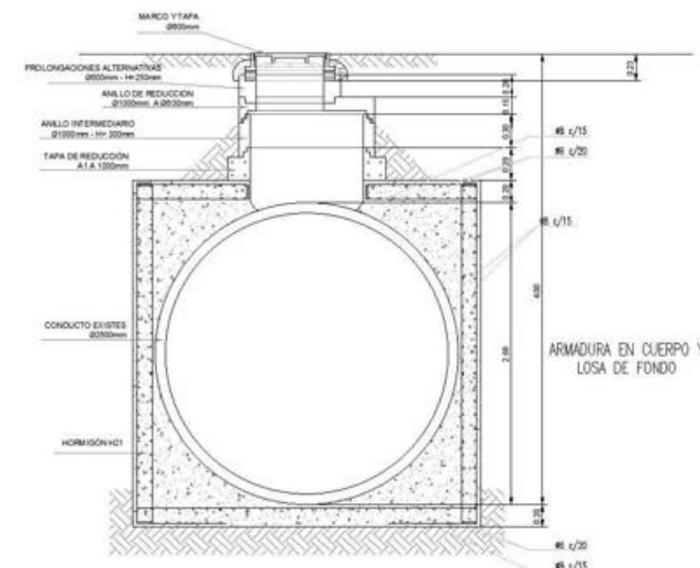
Arriba: Detalle cámara de inspección cloacal Abajo: | Boca de registro cloacal.
