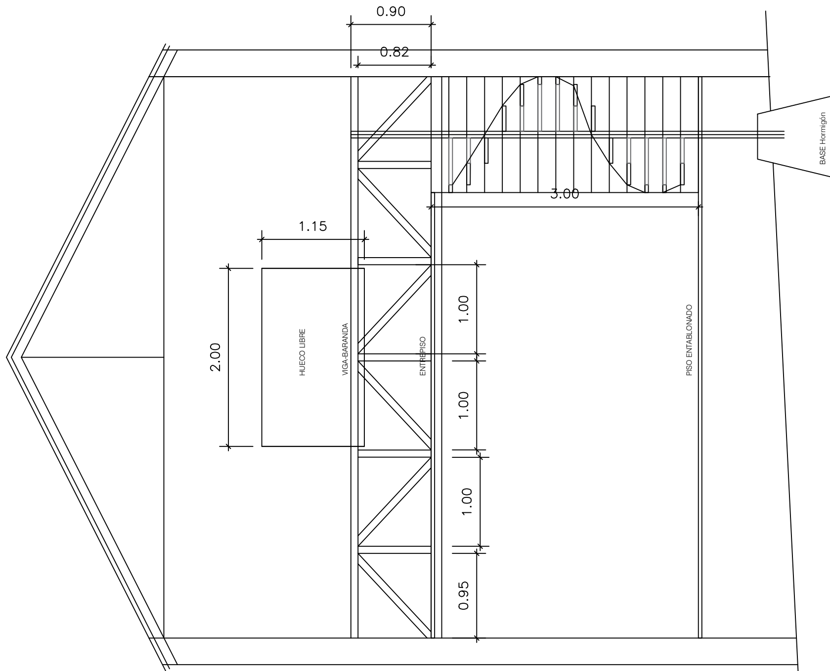
Corte Transversal
